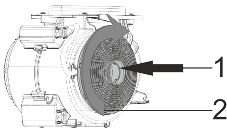
Απεικ. 5: ΦΙΛΤΡΟ ΑΝΘΡΑΚΑ
